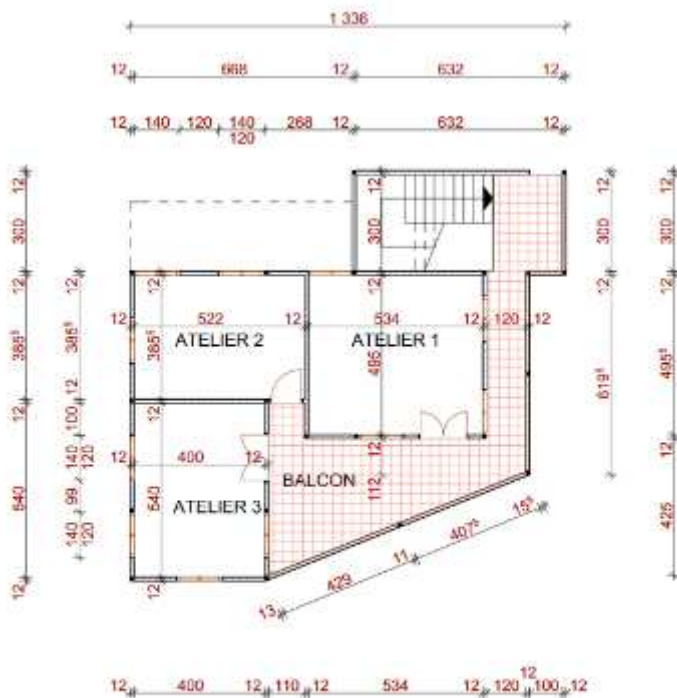
LIBRAIRIE (CENTRE POUR LA FAMILLE) VUE EN PLAN R+1 + COTATIONS ECHELLE 1/100
