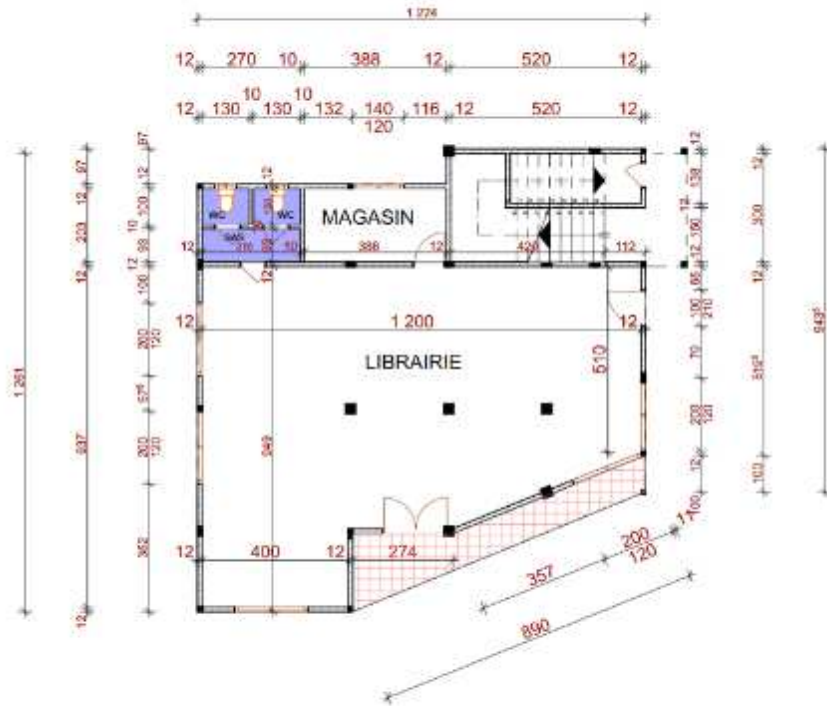
LIBRAIRIE (CENTRE POUR LA FAMILLE) VUE EN PLAN RDC + COTATIONS ECHELLE 1/100
